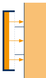
Такая конструкция подсветки разрешена на всех типах зданий.
